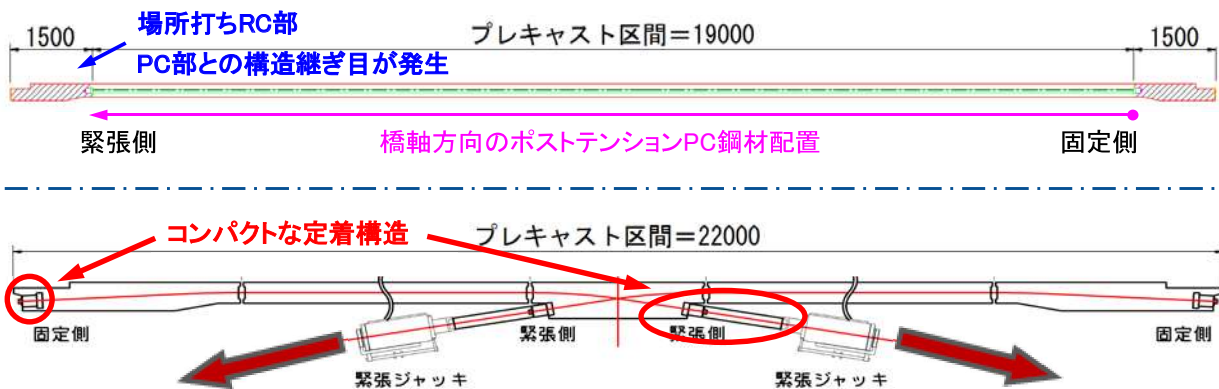
PC 鋼材の配置方法比較(上段:従来工法、下段:交差定着によるオールプレキャスト化)
