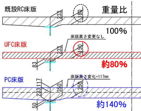
床版の厚さおよび重量の比較
